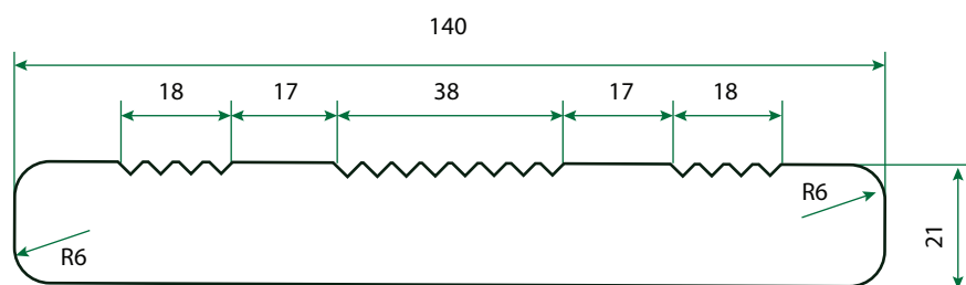
SECCION TRANSVERSA
